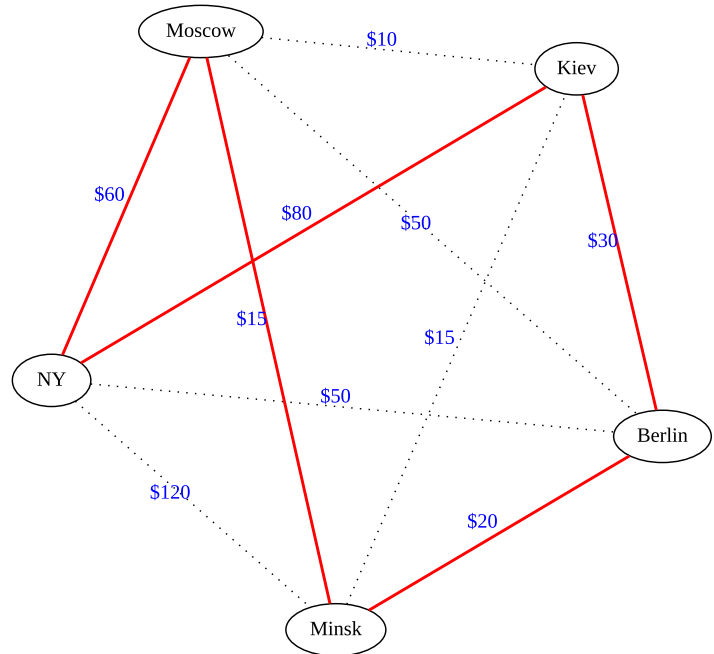
Рис. 1.1: Работа алгоритма 6 «TSP-перебор»
