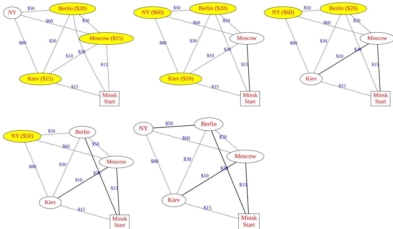
Рис. 1.4: Иллюстрация работы алгоритма 9 «MST Прима»
