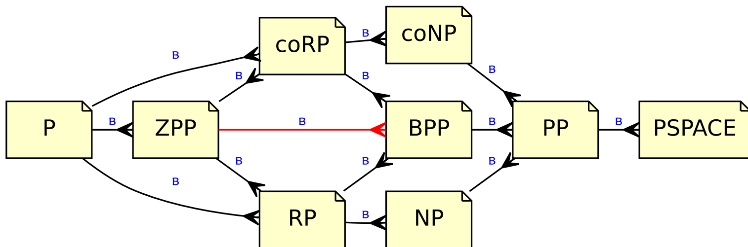
Рис. 6.13: Вероятностные классы сложности: ZPP , RP , BPP , PP
