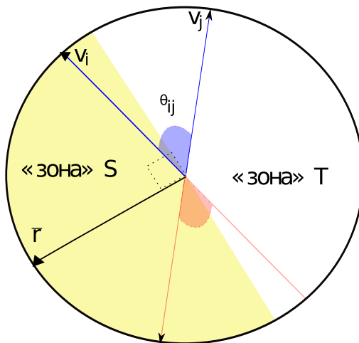
Рис. 4.6: Вектора в вероятностном округлении «MAX-CUT»
