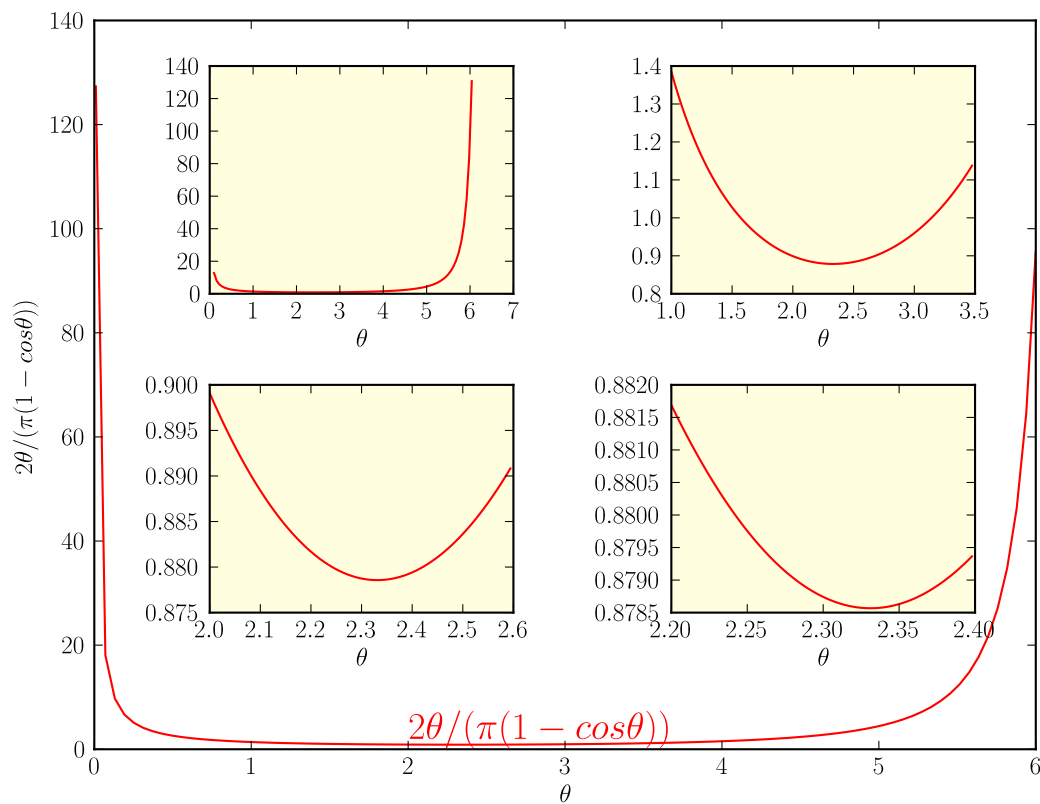
Рис. 4.5: График функции \frac{2\theta}{\pi(1-\cos\theta)}
