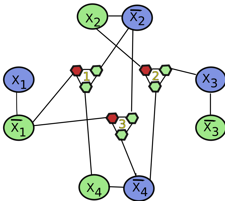
Рис. 6.8: Отображение выполнимой КНФ на граф
