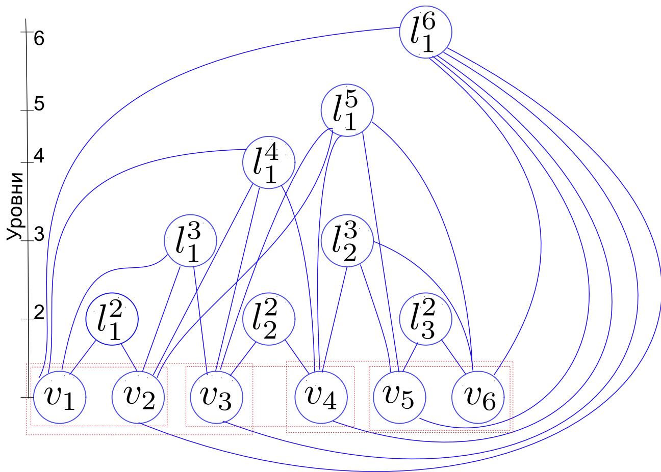
Рис. 2.1: «Плохой» граф для жадного алгоритма вершинного покрытия
