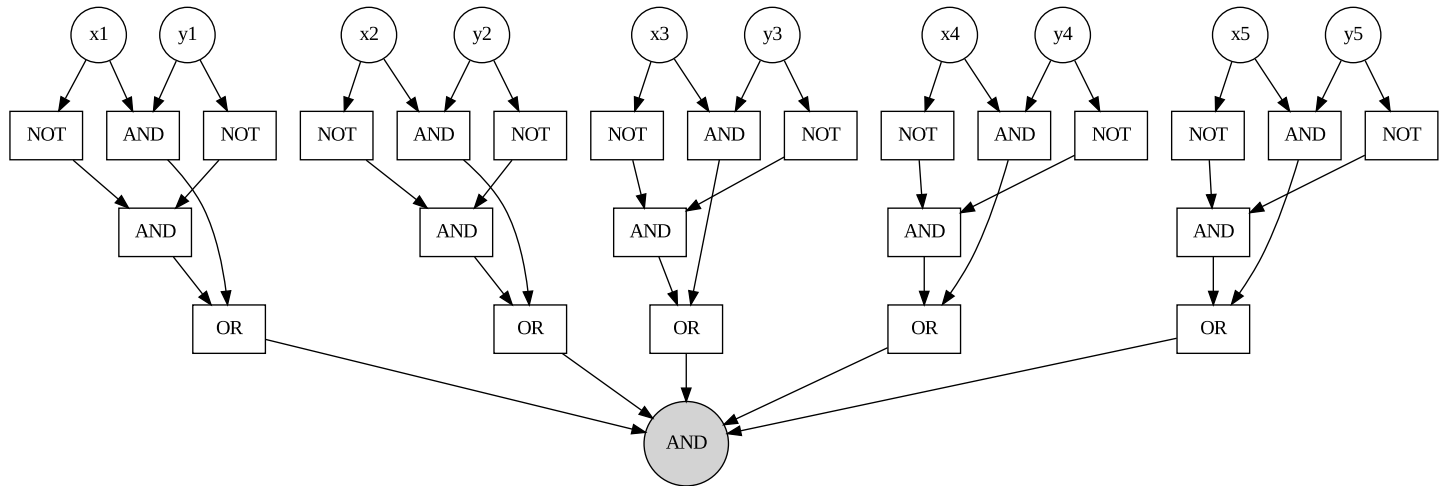
Рис. 6.17: Пример схемы: сравнение двух строк
