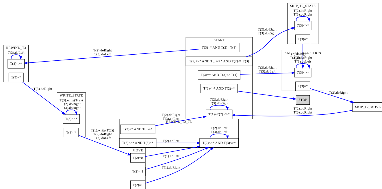
Рис. 6.6: Трехленточная универсальная МТ для одноленточных МТ
