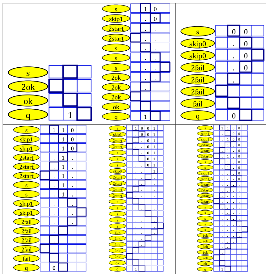
Рис. 6.5: Выполнение МТ «Количество 0 и 1 равно?»
