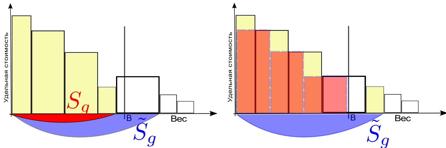
Рис. 2.6: Наборы S_g и \tilde{S}_g в «жадном» алгоритме для «рюкзачка»
