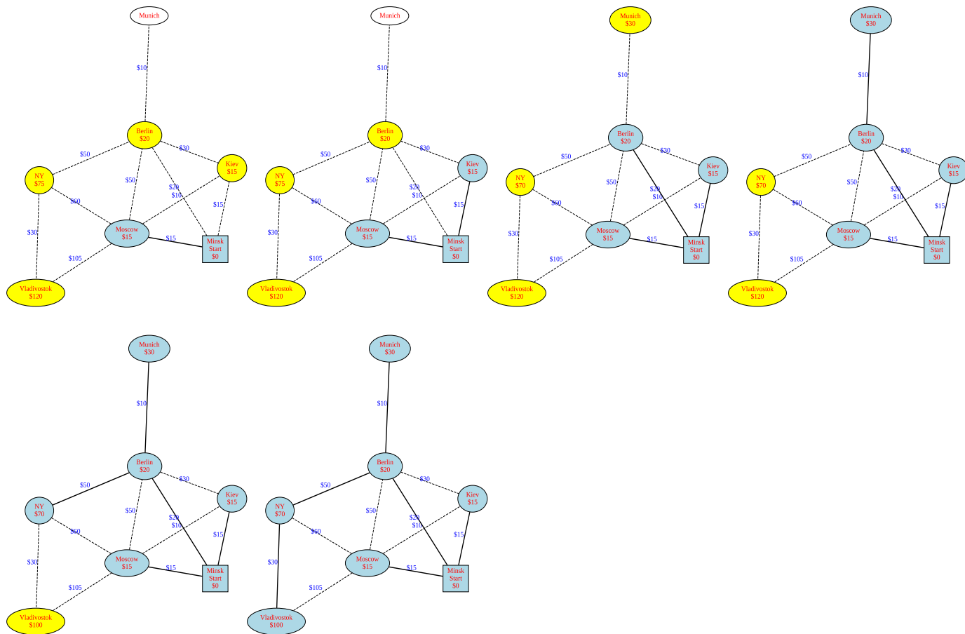
Рис. 1.2: Работа алгоритма 7 «Дейкстры»
