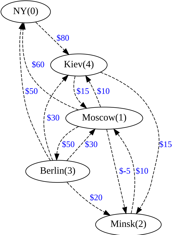
Рис. 1.3: Иллюстрация работы алгоритма 8 «Флойда – Уоршолла»
