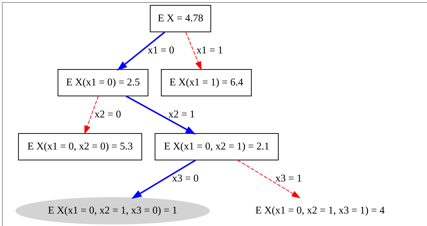
Рис. 5.1: Дерандомизация на основе минимизации оценок математического ожидания
