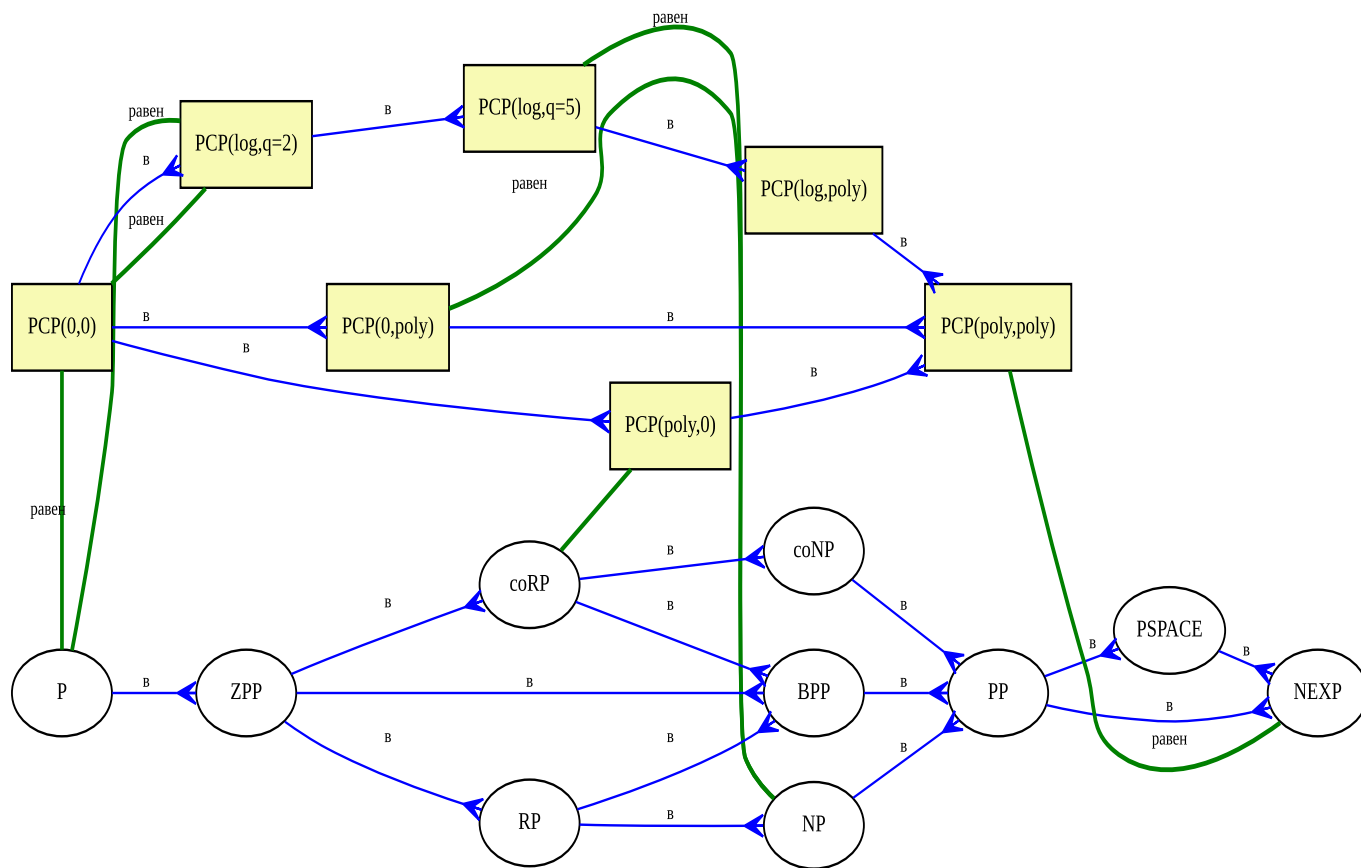
Рис. 6.19: Иерархия некоторых классов сложности
